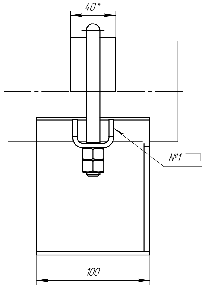
Det. poz. 2 (1:1)
