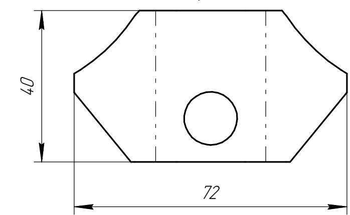
Det. poz. 7 (1:1)
